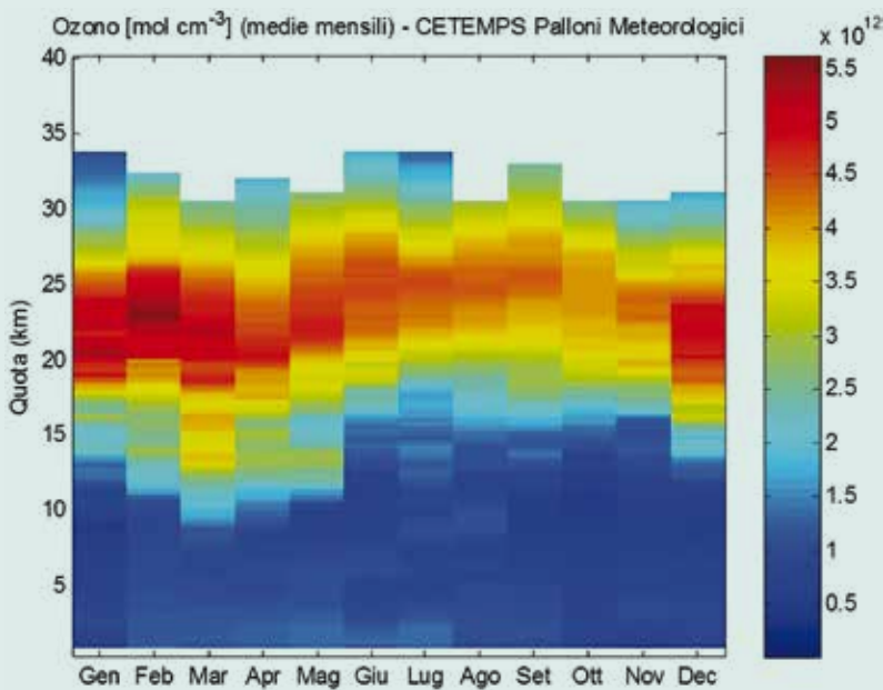
Figura 6.09 Ozono [ \text{mol cm}^{-3} ] (medie mensili) Fonte CETEMPS
